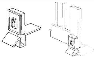
MEA1 Dispositivo per apertura a 360°
