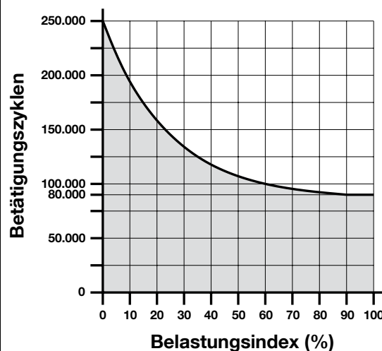
SCHAUBILD A
